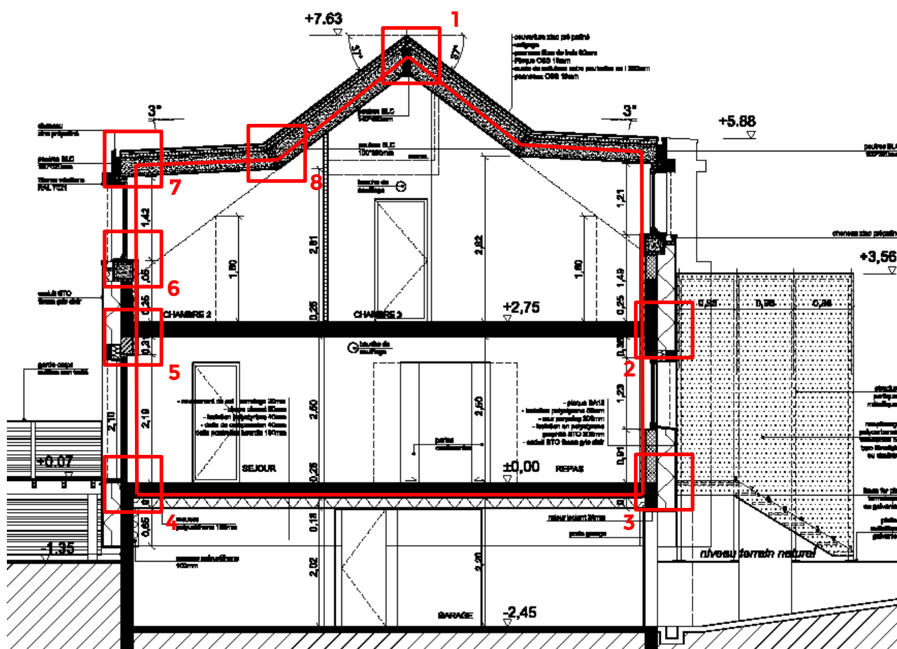
Figure 5 : Exemple de coupe [Karawitz Architecture]
