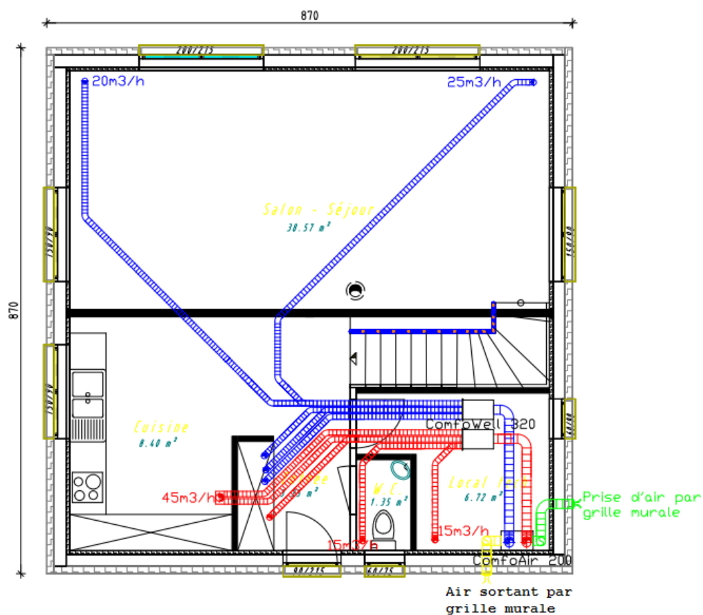
Figure 10 : Exemple de plan de ventilation (Extrait)
